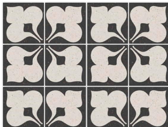
Muon G.156
